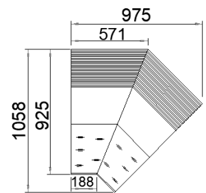
ZITA MINI 45°I
