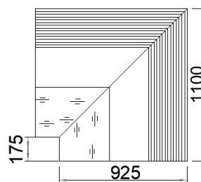
ZITA MINI 90°I
